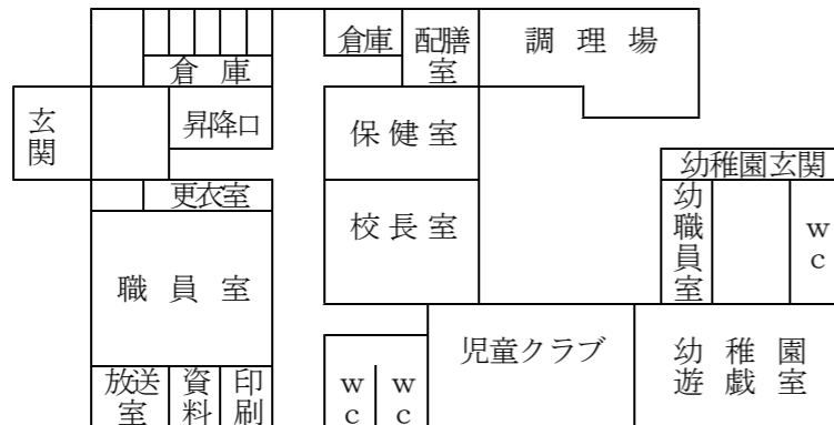
1階平面図
